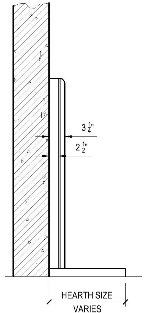
LEFT SIDE
